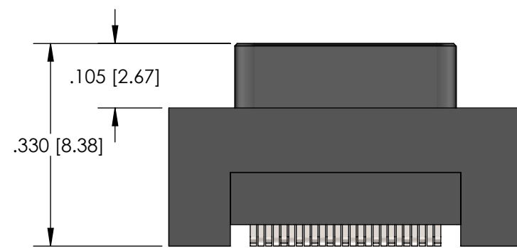
PLUG (PINS)
